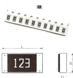
resistenze SMD
